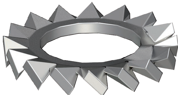
Vějířová podložka podle DIN 6798, tvar A.
