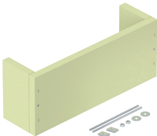
Křemičitan vápenatý
