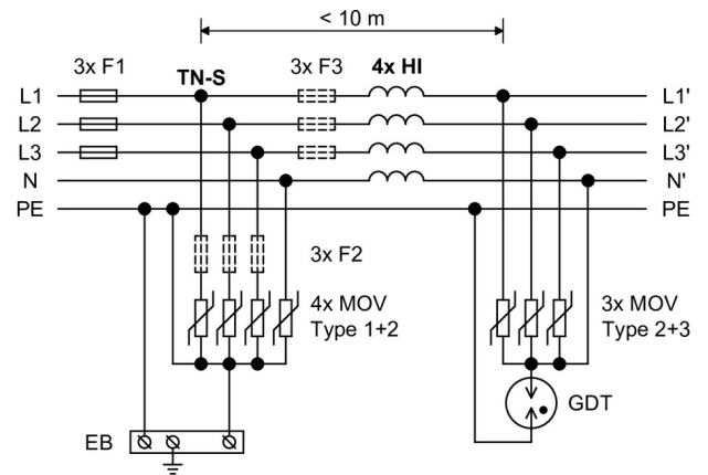
Aplikační schéma zapojení (instalace)
