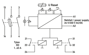
Anschlussschema
