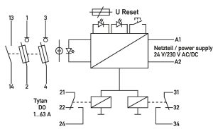
Anschlussschema
