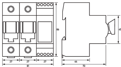
Maßzeichnung Gruppenansicht
