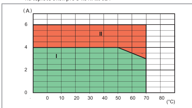
L 34-1 - Zatížitelnost výstupu - závislost výstupního proudu na teplotě okolí pro 34.81.7...9024
