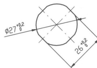
Montážní otvor
