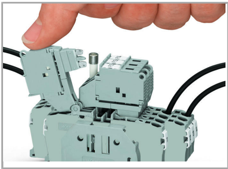
Sicherungsklemme mit schwenkbarem Sicherungshalter
