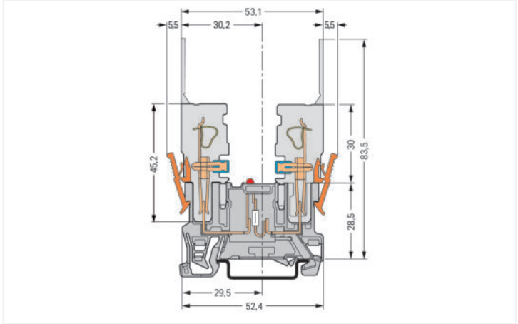
Základní svorka s LED signalizací
