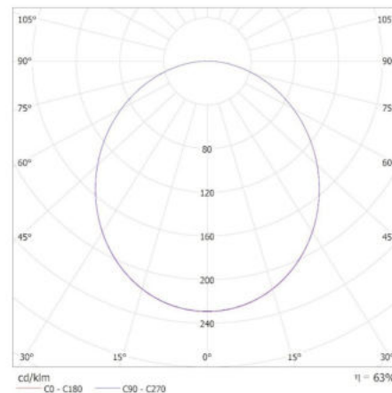
KANLUX S.A. (kat 38786) BENO 24-30W CCT-O W 24W / Krzywa rozsyłu światła (biegunowo)
