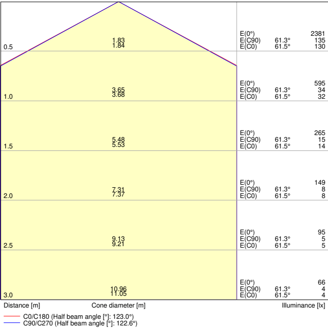
SF SLIM SQ S 200 P 19W 830 IP65 WT
