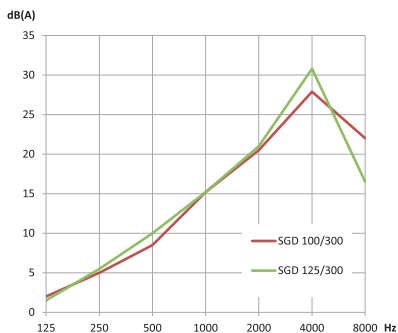
SGD – tlumič vsuvný, vložný útlum
