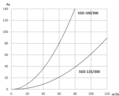
tlaková ztráta (typické hodnoty)
