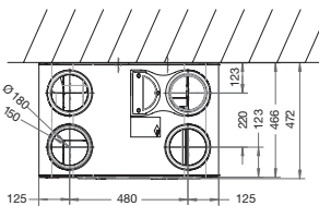
pohled shora – připojovací hrsla
