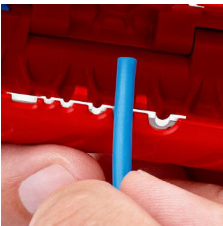
90 22 02 SB: Praktická pomůcka pro polohování usnadňuje vkládání jednotlivých vodičů pro odizolování
