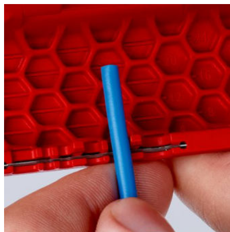
90 22 02 SB: Nastříhaná délková stupnice pro rovnoměrné odizolování v jednotné délce, čitelná pro praváky i leváky
