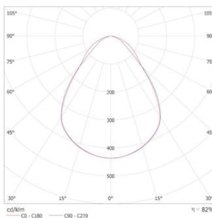
KANLUX S.A. (kat 33179) BLINGO TUN 48W 6060 NW / Krzywa rozsyłu światła (biegunowo)
