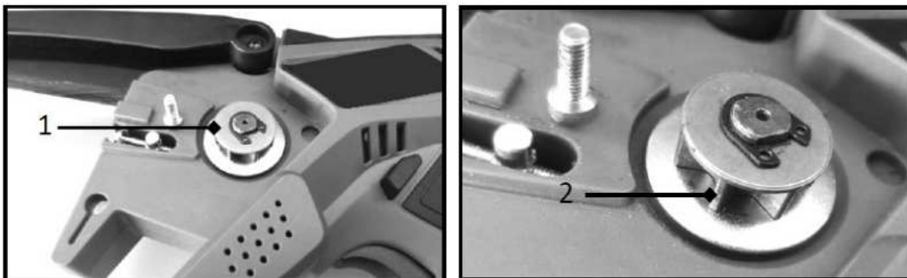
1. Wałek zębaty; 2. Elementy sprawdzone pod kątem zużycia
