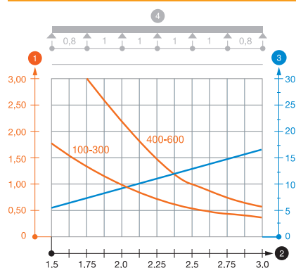
Zatěžovací diagram kabelového žlabu DKS 60 VA
