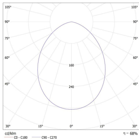
KANLUX S.A. (kat 33360) AQILO IP65 DSO-W + IQ-LED / LDC (Polar)
