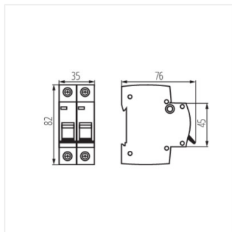
KMB6-B25/2
