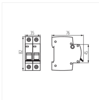
KMB6-B63/2
