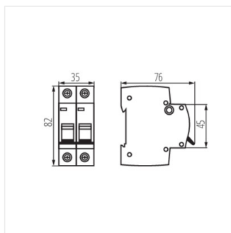
KMB6-B6/2
