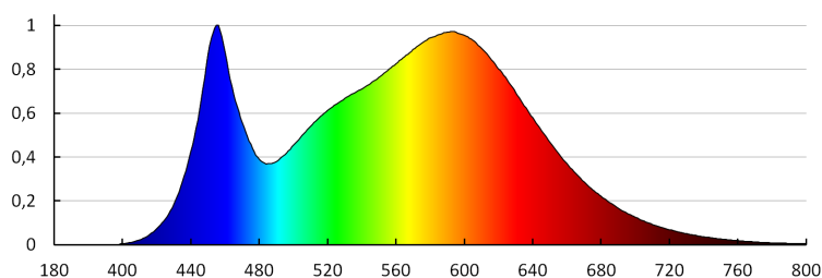
MILEDO (kat 31184) GRUN V3 LED-70-B / LDC (Polar)
