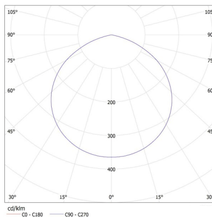
MILEDO (kat 31184) GRUN V3 LED-70-B / LDC (Polar)
