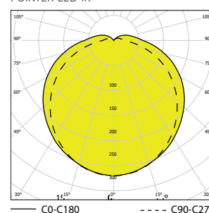
POINTER-LED-1R
