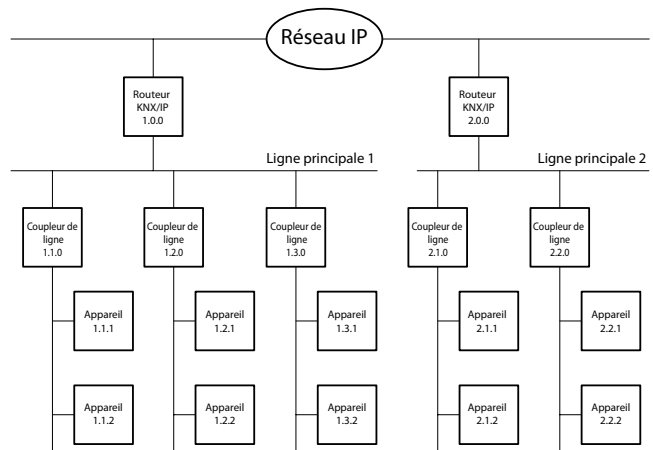
Fig. 2 : Routeur IP jouant le rôle de coupleur de zone
