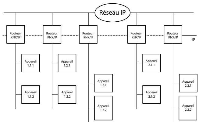
Fig. 3 : Routeur IP jouant le rôle de coupleur de ligne
