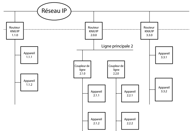
Fig. 1 : Routeur IP jouant le rôle de coupleur de ligne/zone
