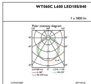
IFPC1_WT060CL600LED18S840
