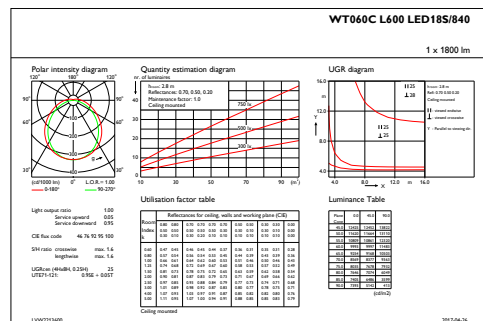
IFGU1_WT060CL600LED18S840
