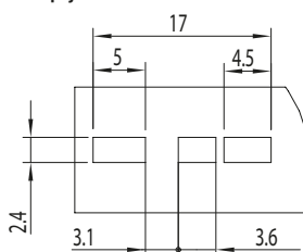
Vzor pájení PCB
