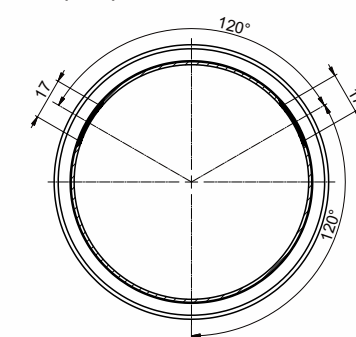
B-B (1 : 1)
