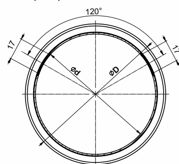
A-A (1 : 1)
