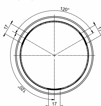
B-B (1 : 1)
