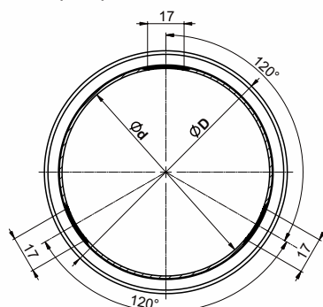
A-A (1 : 1)
