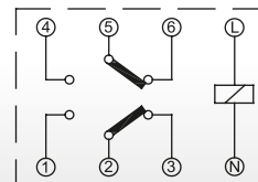
Schéma zapojení
