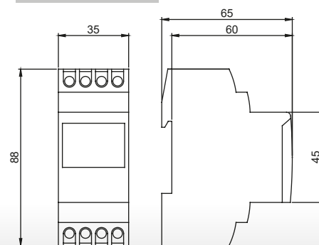
Rozměry
