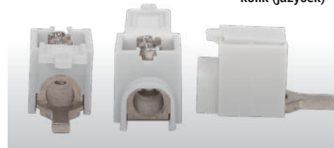
2 šrouby pro utažení vodiče (vhodné pro měděné vodiče do průřezu 25 mm 2 )
