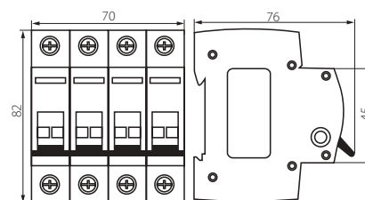
Rozměry / Rozmery
