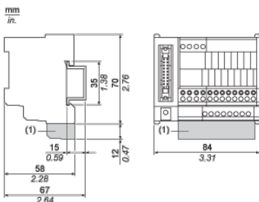
(1) ABE7BV10 / ABE7BV10E
