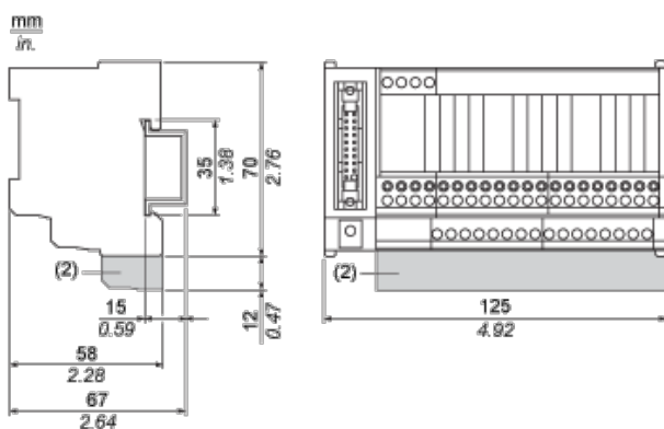
(2) ABE7BV20 / ABE7BV20E
