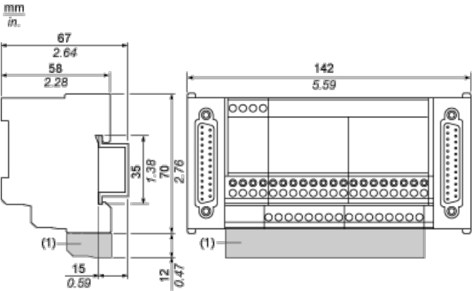
(1) ABE7BV20
