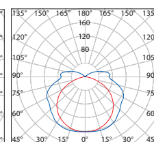
DUST EVG PC 2 × 58W
