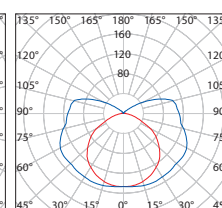
DUST EVG PC 1 × 58W
