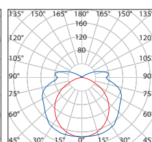
DUST EVG PC 2 × 36W
