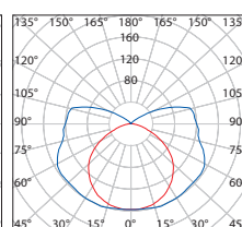
DUST EVG PC 1 × 36W
