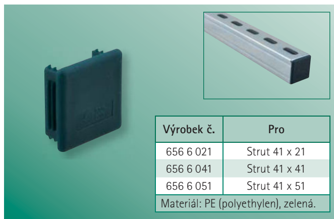
BIS Strut Koncové ucpávky
