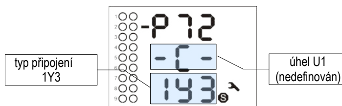
Obr. 4.24: Typ jednofázového zapojení 1Y3 a úhel U1
