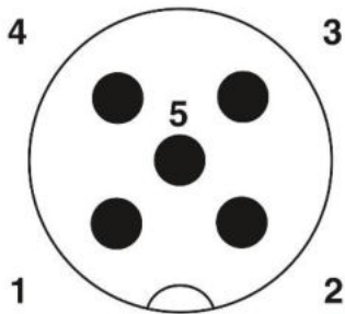
Pin assignment M12-plug, 5-pol, A-codiert
