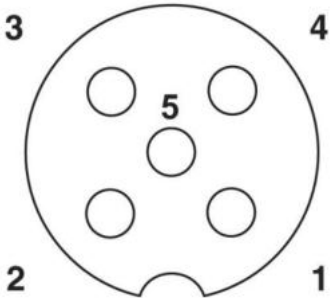
Pin assignment M12-jack, 5-pol, A-codiert
