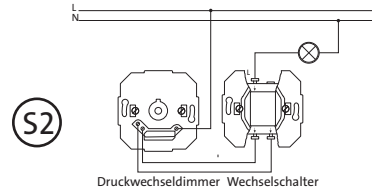
Drukwechseldimmer Wechselschalter
