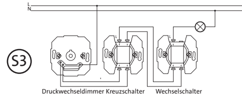
Drukwechseldimmer Kreuzschalter Wechselschalter
