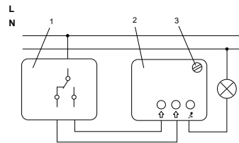
Wechselschaltung - Wisselschakeling - Circuit va-et-vient
