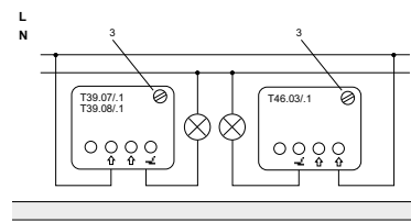
Ein-Ausschaltung - 1-polige schakeling - Circuit unipolaire
