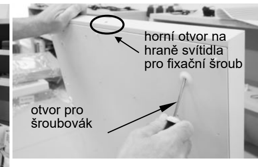
PO ZAVŘENÍ SVÍTIDLA ZAŠROUBOVAT A VLOŽIT BÍLOU KRYTKU DO FIXAČNÍHO OTVORU
