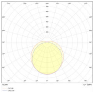
DP 3TH 1500 E 65W 857 IP65 GY
