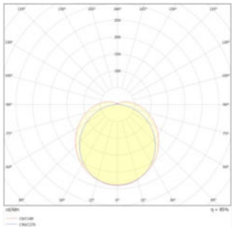
DP 3TH 600 E 17W 865 IP65 GY
