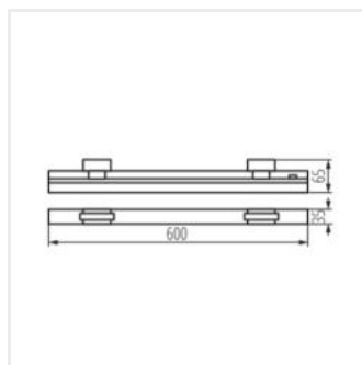
LTL-E 15W-60-CCT-B
