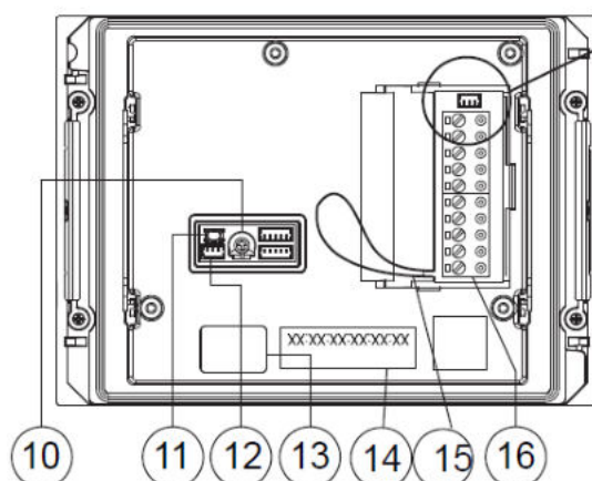
ZADNÍ POHLED 1083/39
