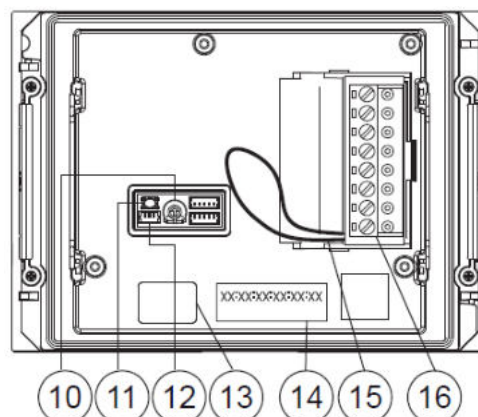
ZADNÍ POHLED 1083/38 A 1083/48
