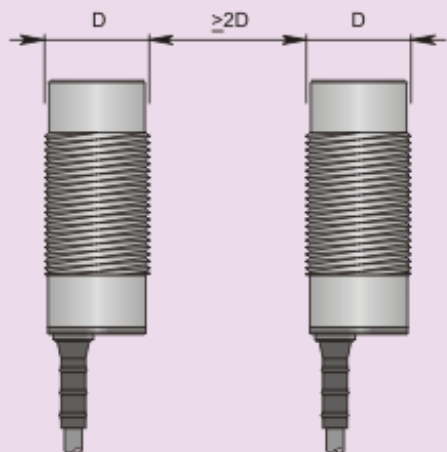
Montaggio affiancato
