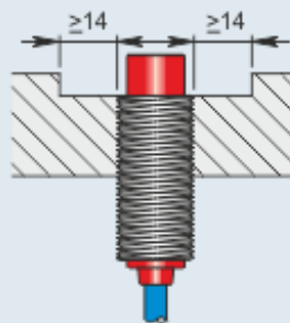
Montaggio sporgente
