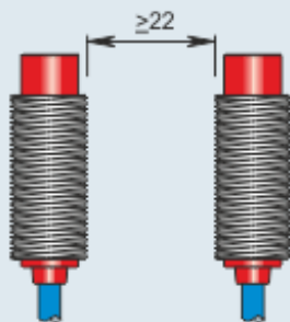
Montaggio affiancato
