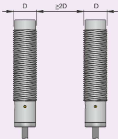
Montaggio affiancato
