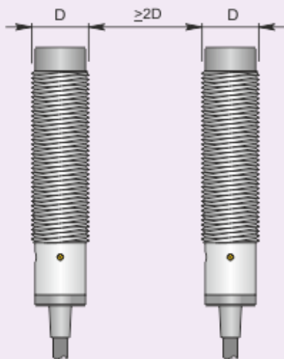
Montaggio affiancato
