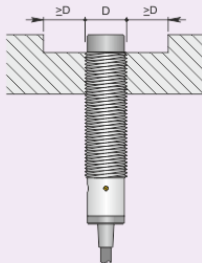
Montaggio sporgente
