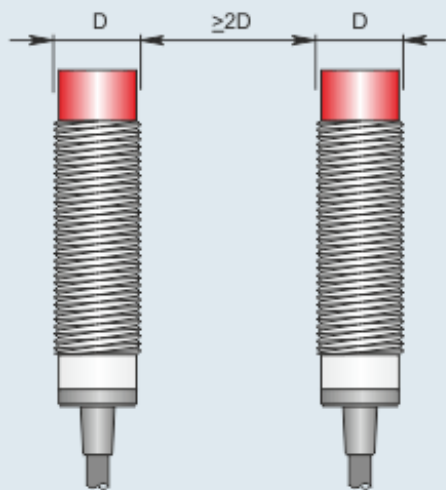
Montaggio affiancato
