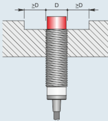
Montaggio sporgente
