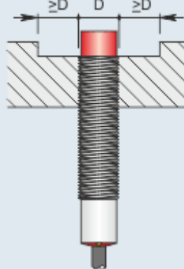
Montaggio sporgente
