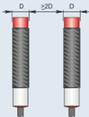
Montaggio affiancato
