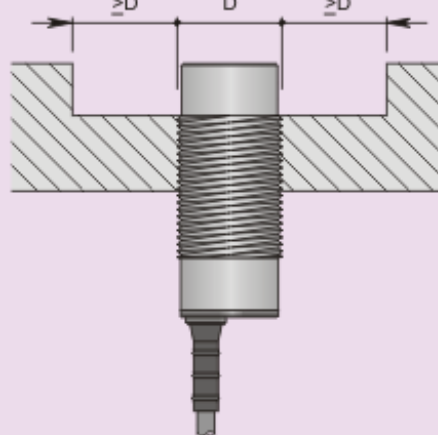
Montaggio sporgente
