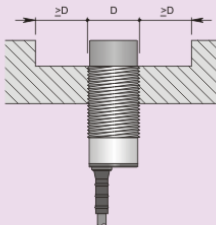
Montaggio sporgente
